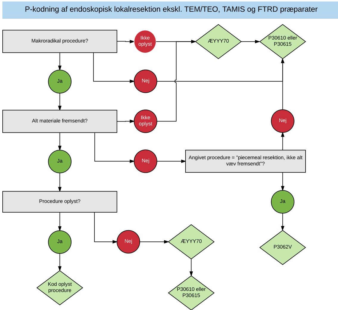
Figur 1 P-kodning flowchart
